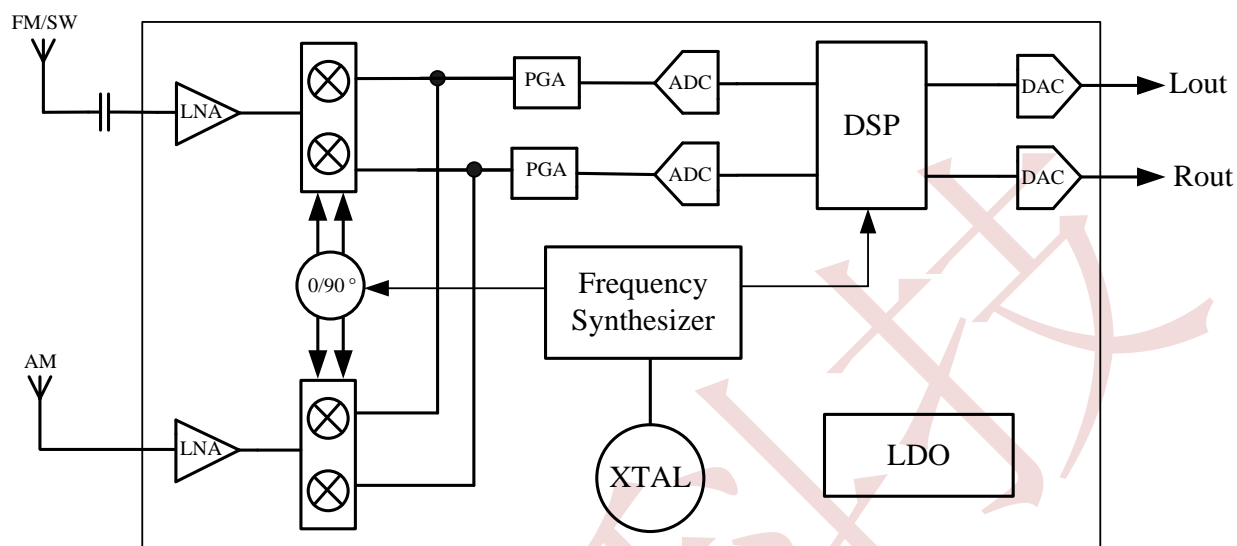
图 1. C9616 功能框图
