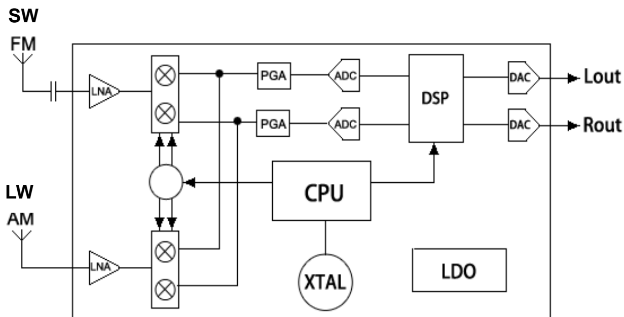
图 1. C9620 功能框图
