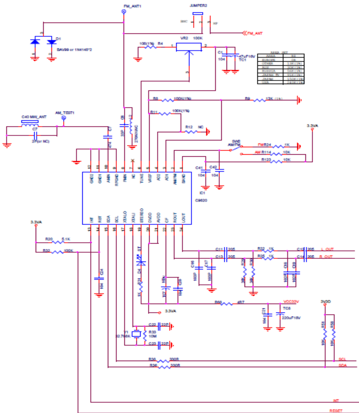
(图 11. 典型应用原理图)
