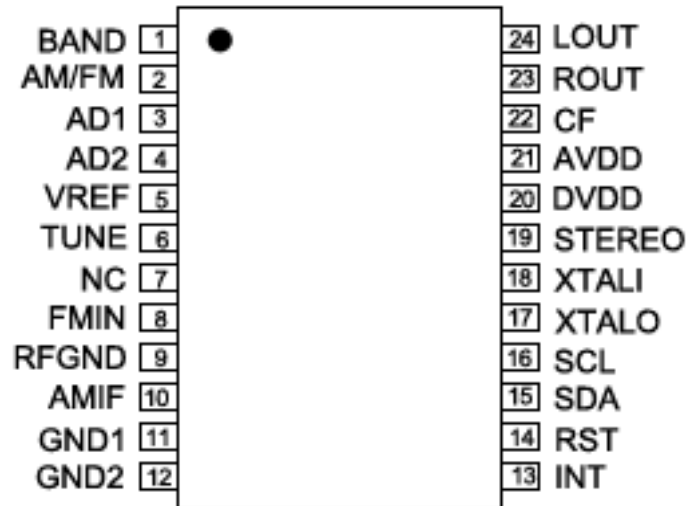
(表 7. CA9620 芯片引脚描述)
