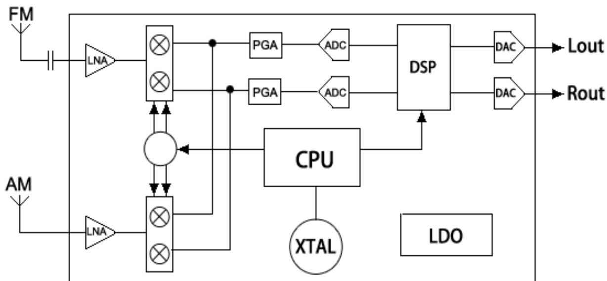
图 1. C9612 功能框图
