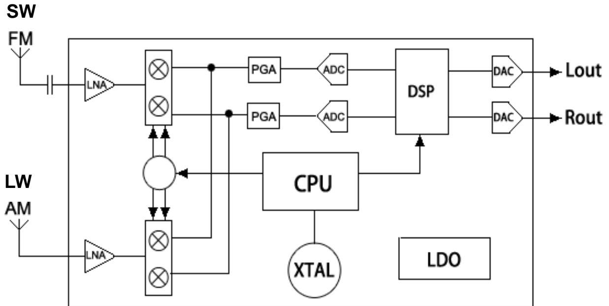
图 1. C9610 功能框图
