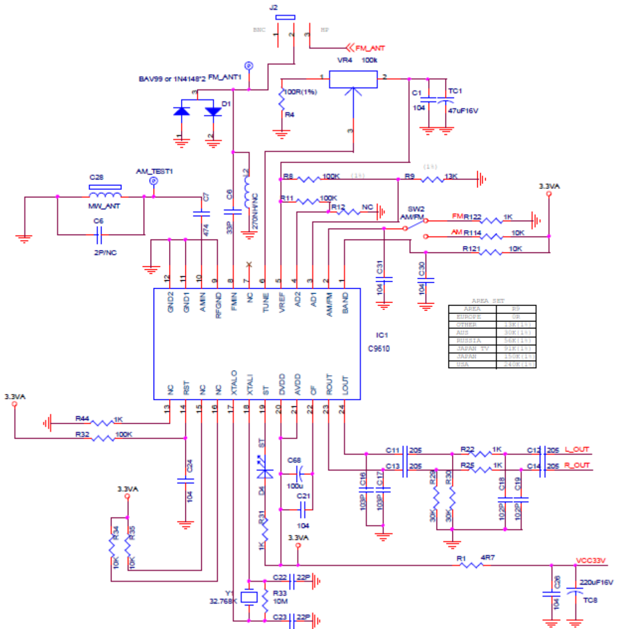
(表 11. 典型应用原理图)
