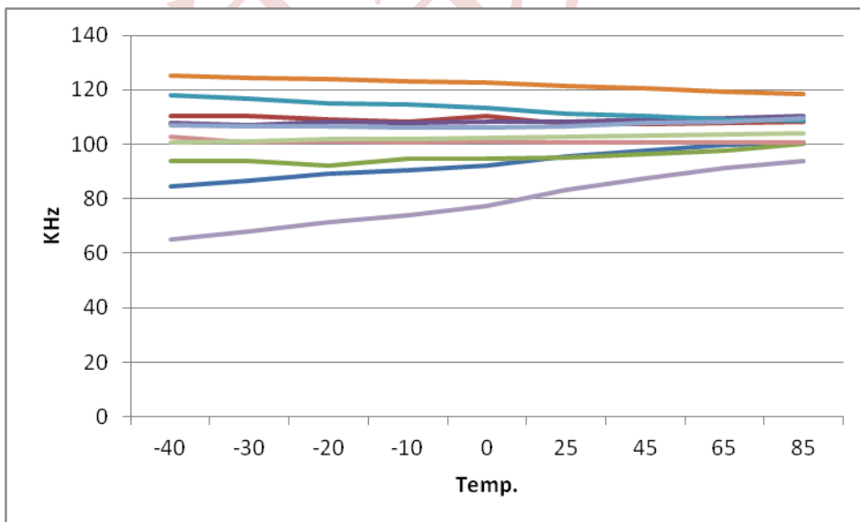
图 23-5-2 IRCL 温度特性曲线图
