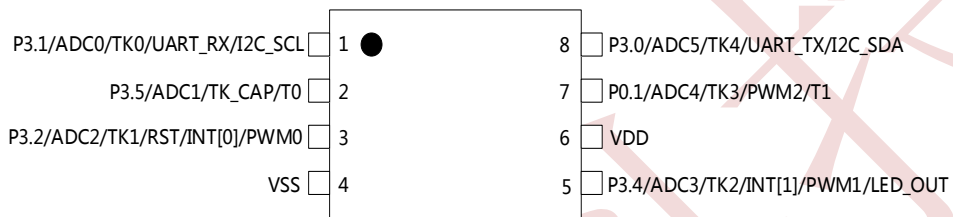
图 5-1-1 SOP8/DFN8 封装图
